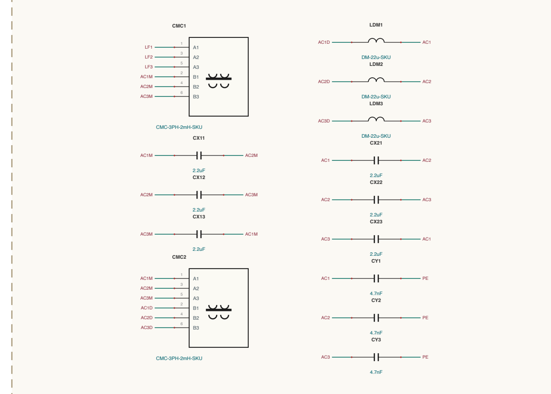
INPUT-EM / EMI-FILTER
