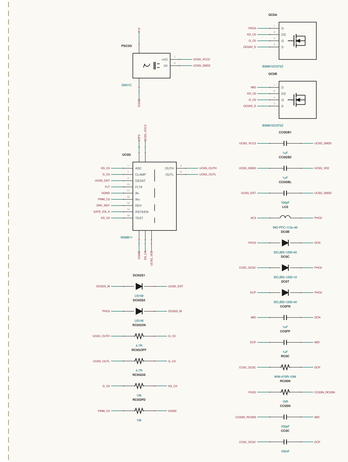
VIENNA-PFC / PHASE-C0
